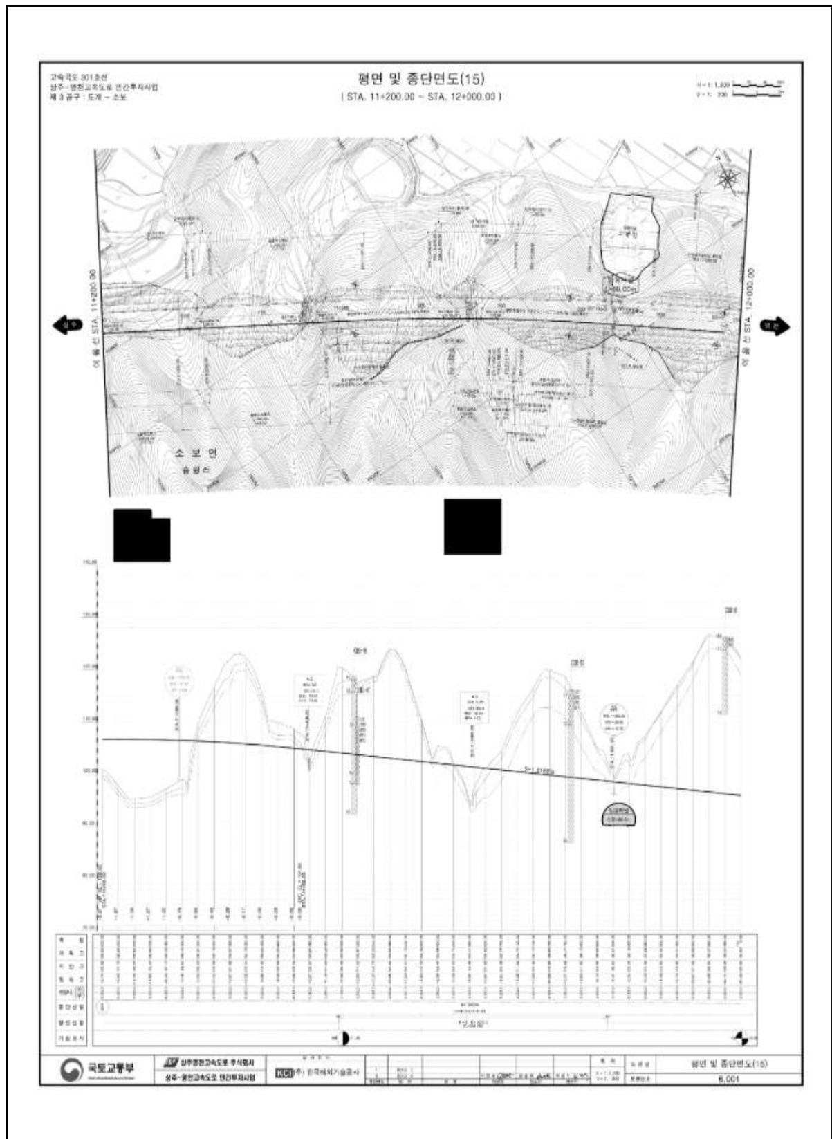
【그림 23.1.4】 평면도
